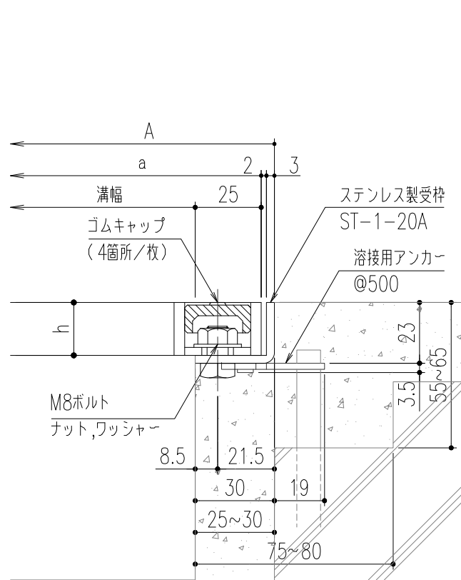
断面詳細図
