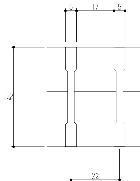
へアリングバー-断面詳細図
