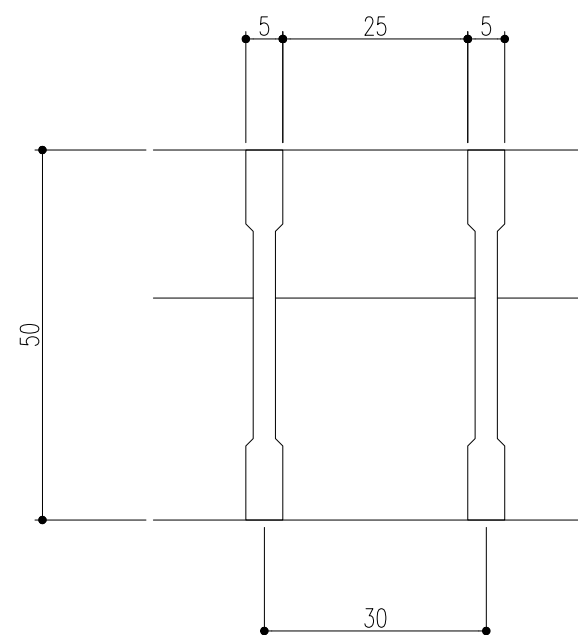
へアリングバー-断面詳細図
