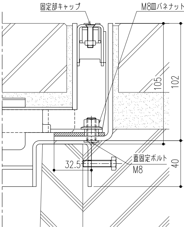
断面詳細図（ボルト固定部） S=1/2
