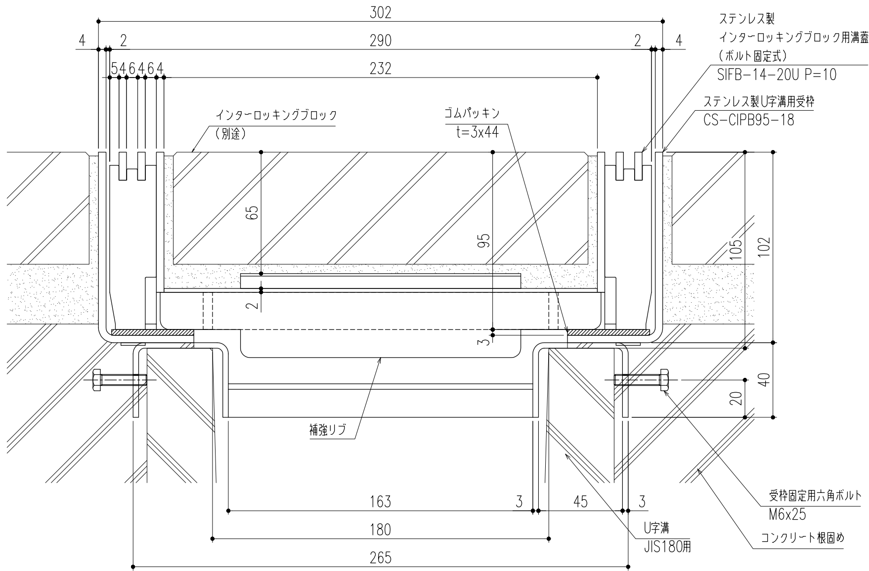
断面詳細図 S=1/2
