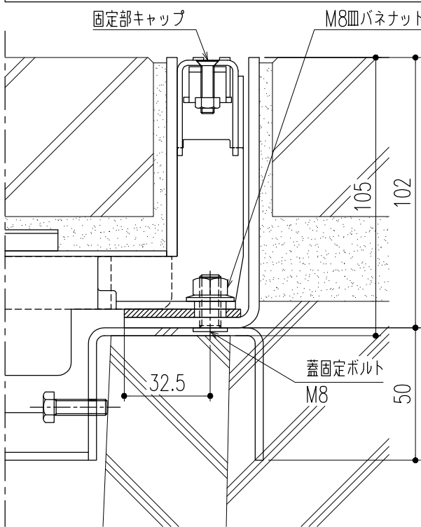
断面詳細図（ボルト固定部） S=1/2
