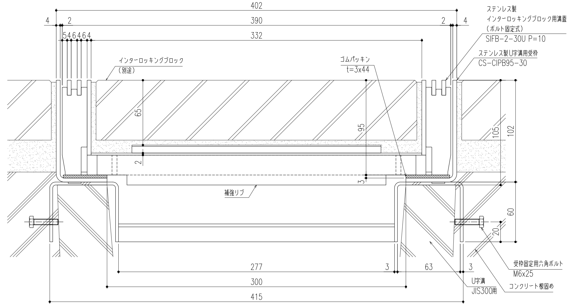
断面詳細図 S=1/2
