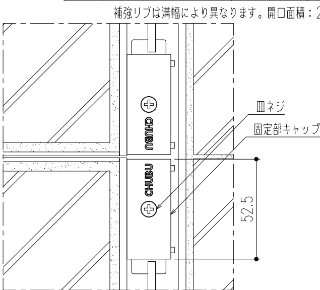
平面詳細図 (ボルト 固定部) S=1/2
