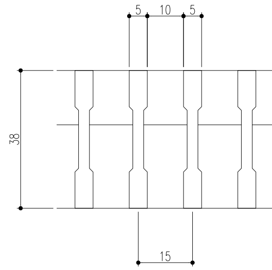
ヘアリングバー-断面詳細図
