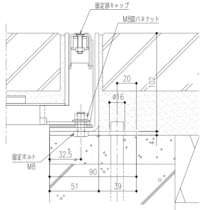
断面詳細図 (ボルト固定部) S=1/2
