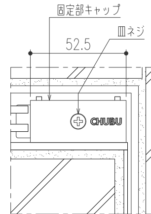
平面詳細図 (ボルト固定部) S=1/2
