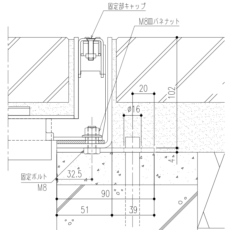
断面詳細図 (ボルト固定部) S=1/2
