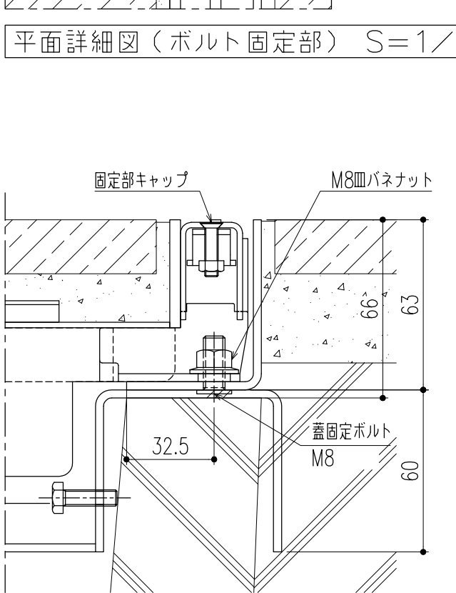
断面詳細図（ボルト固定部） S=1/2
