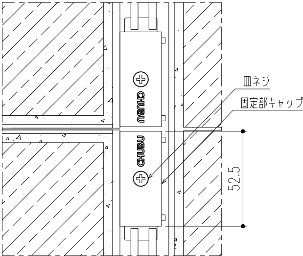
平面詳細図（ボルト固定部） S=1/2
