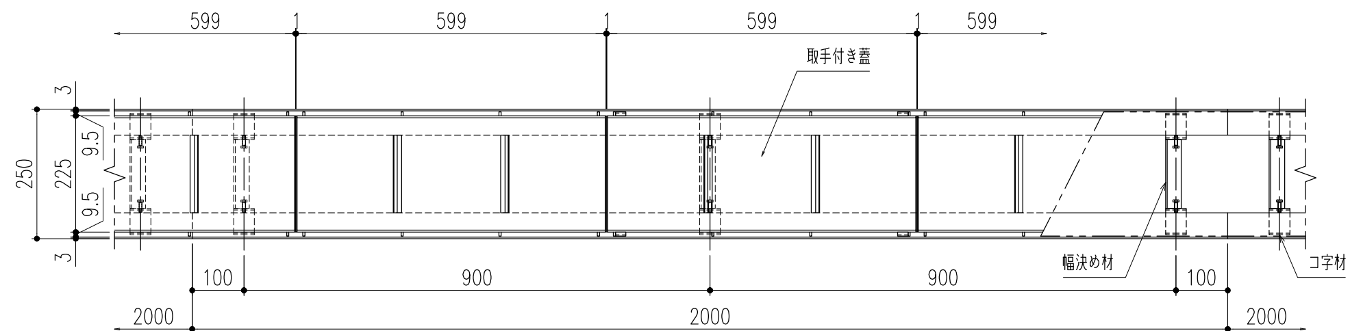
平面詳細図 S=1/10
