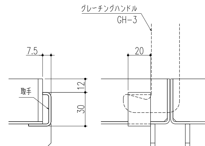
取手部詳細図 S=1/2
