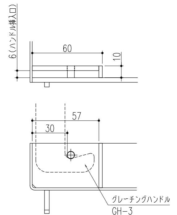
取手部詳細図 S=1/2
