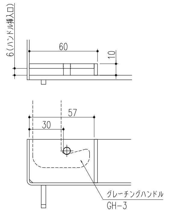
取手部詳細図 S=1/2 ※開閉用として、取手付蓋を10枚に1枚程度ご使用ください。 ＜開閉には専用ハンドルGH-3をご使用ください＞
