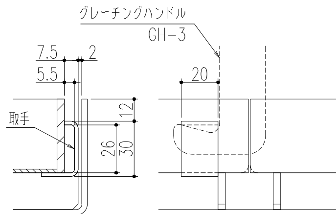
取手部詳細図 (S=1/2)
