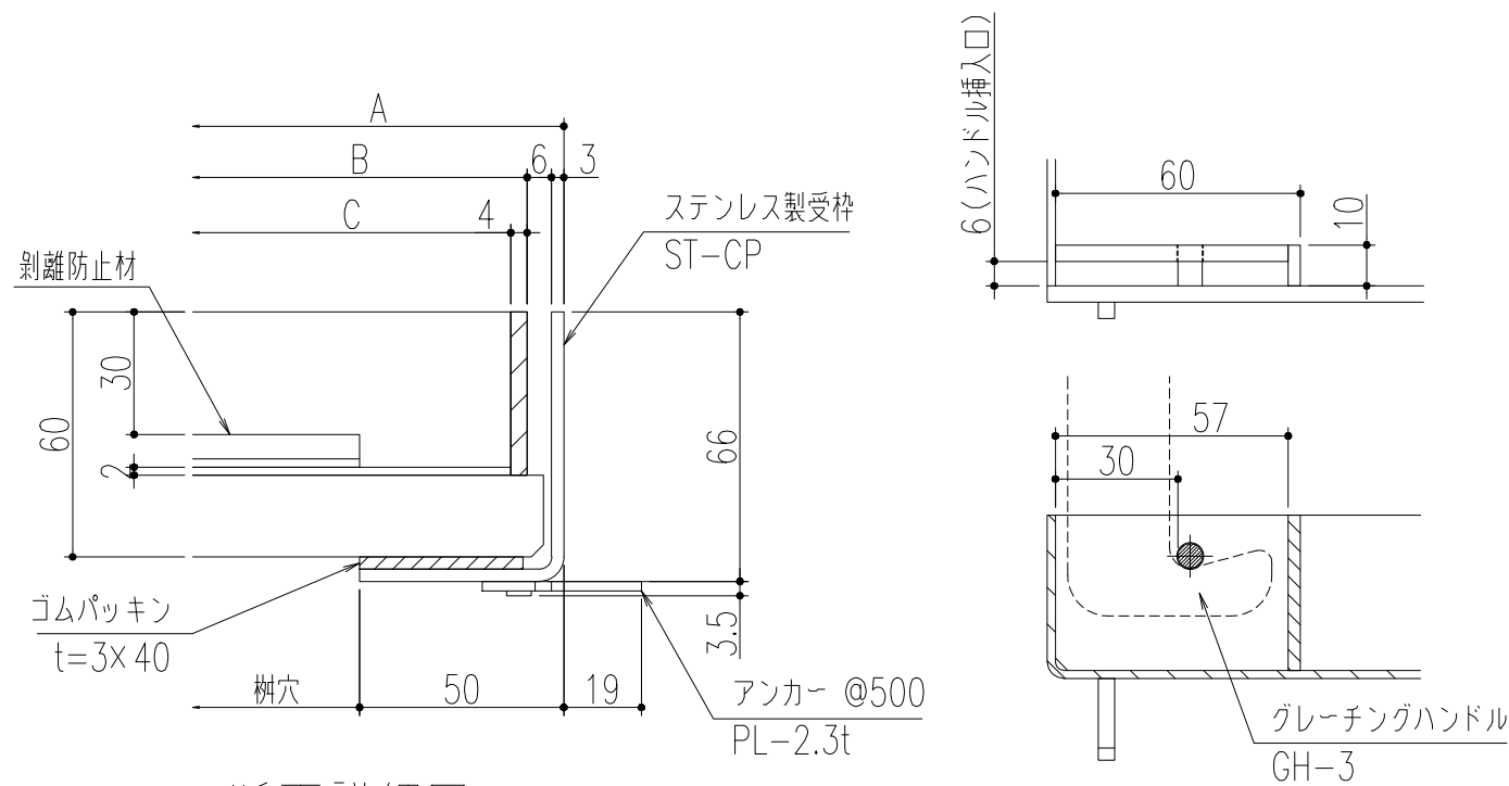
取手部詳細図 (S=1/2)
