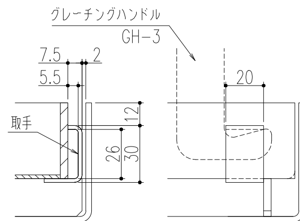
取手部詳細図 (S=1/2)
