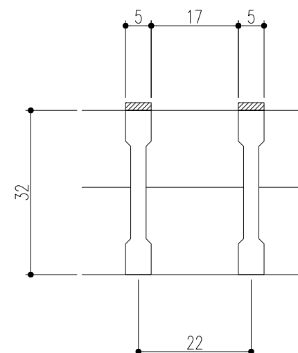
へアリングバー断面詳細図
