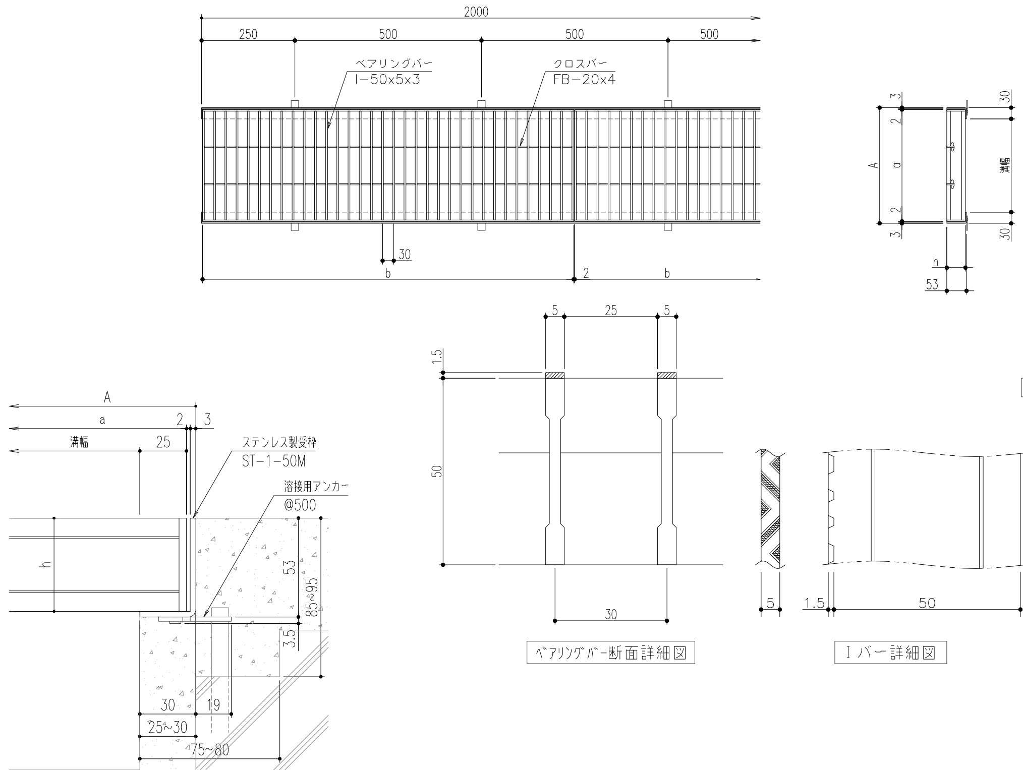
断面詳細図
