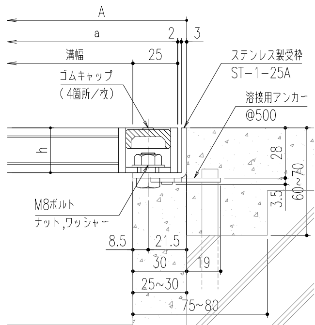
断面詳細図
