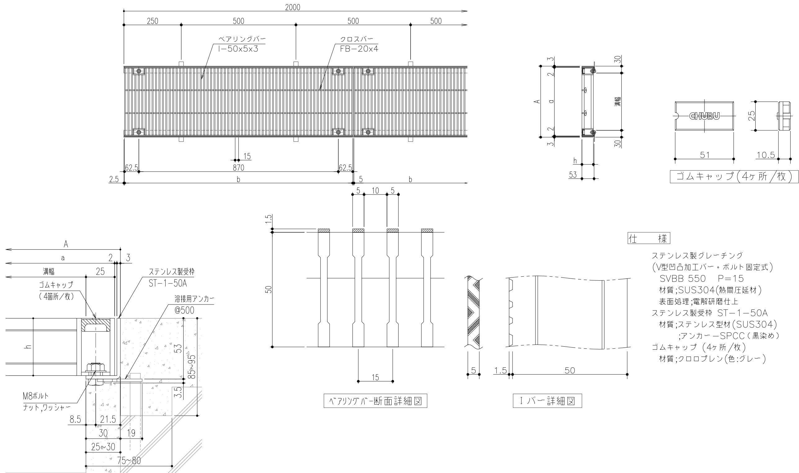
断面詳細図
