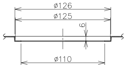
トラップ取付詳細図 S=1/3
