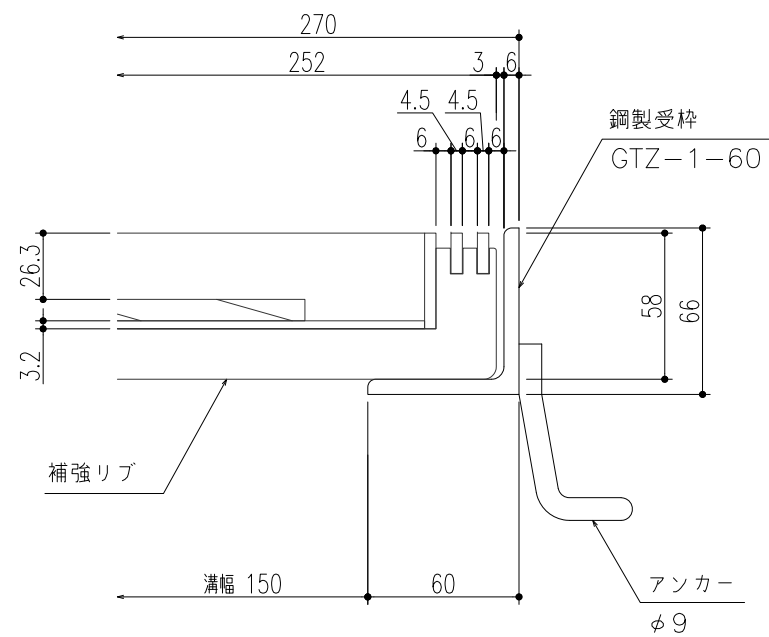
断面詳細図 S=1/3
