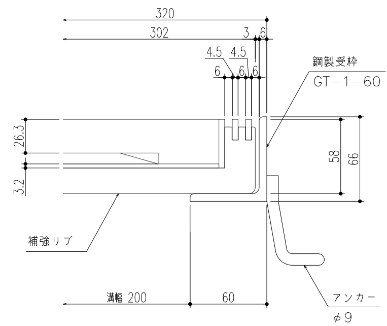
断面詳細図 S=1/3
