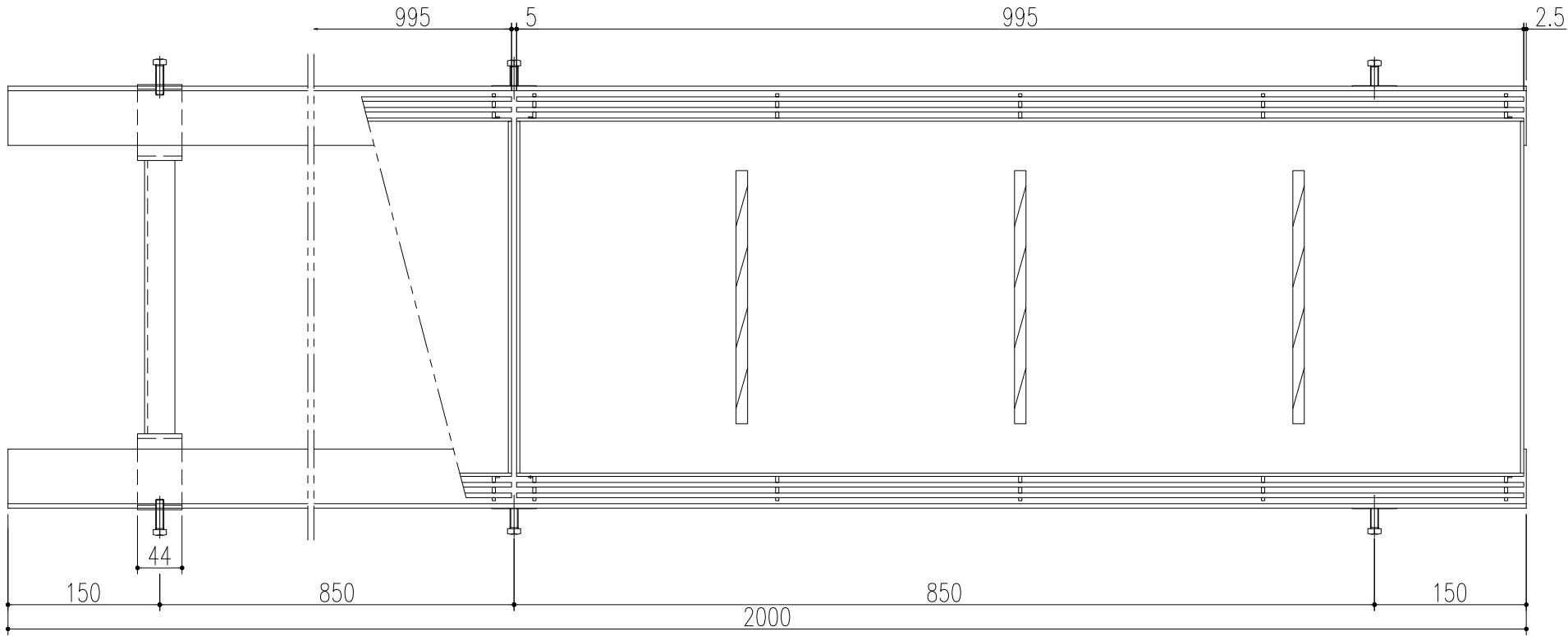
平面詳細図 S=1/6
