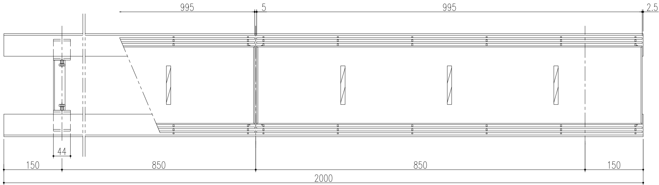
平面詳細図 S=1/6
