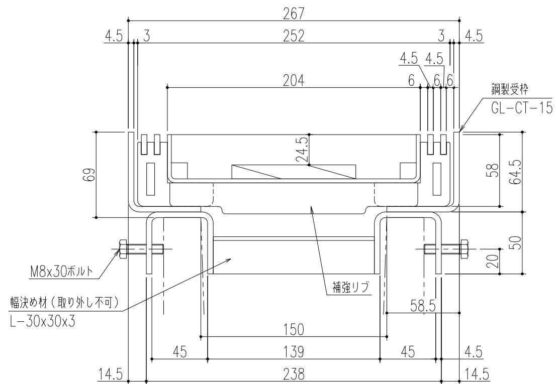
断面詳細図 S=1/3
