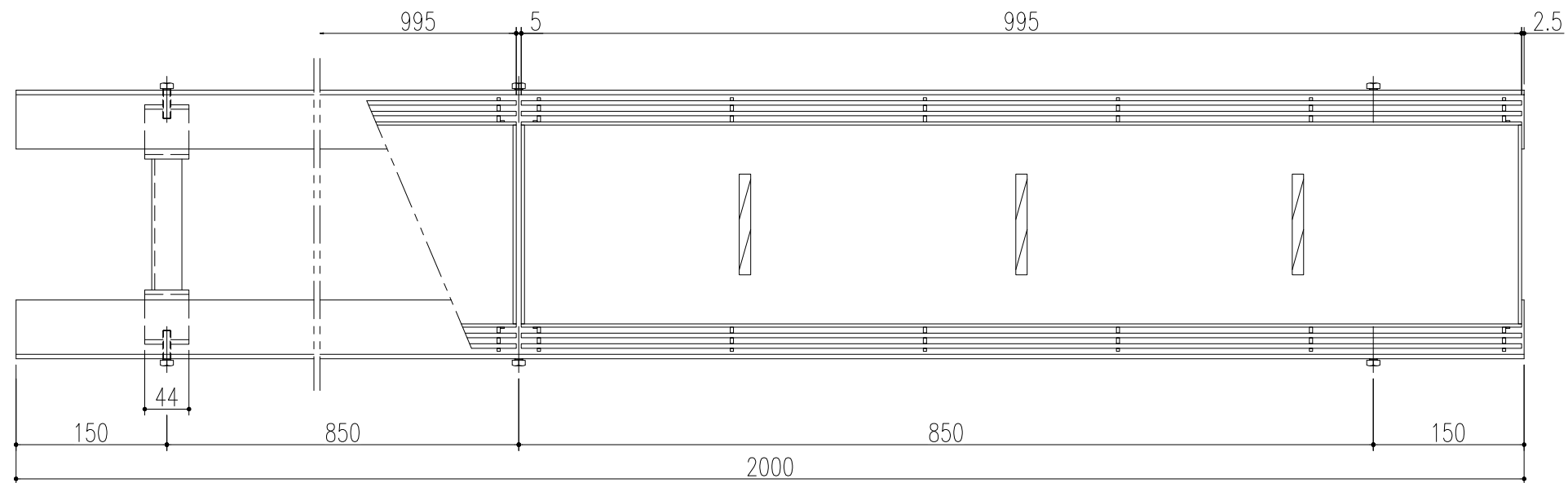
平面詳細図 S=1/6
