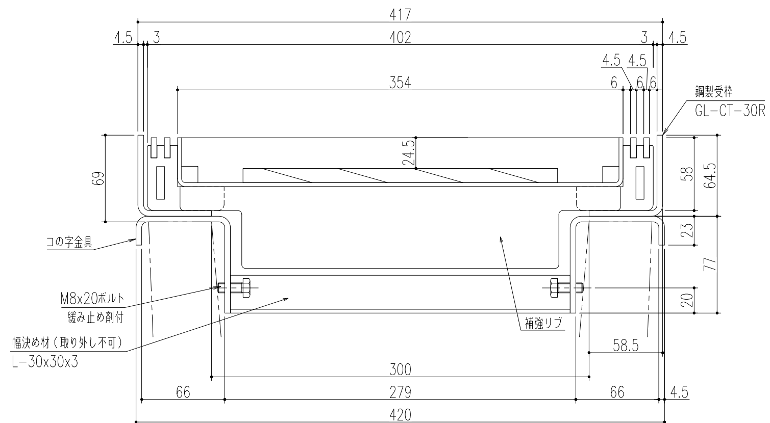
断面詳細図 S=1/3
