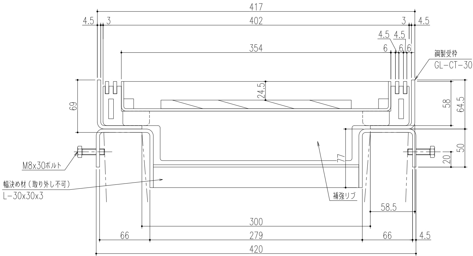
断面詳細図 S=1/3
