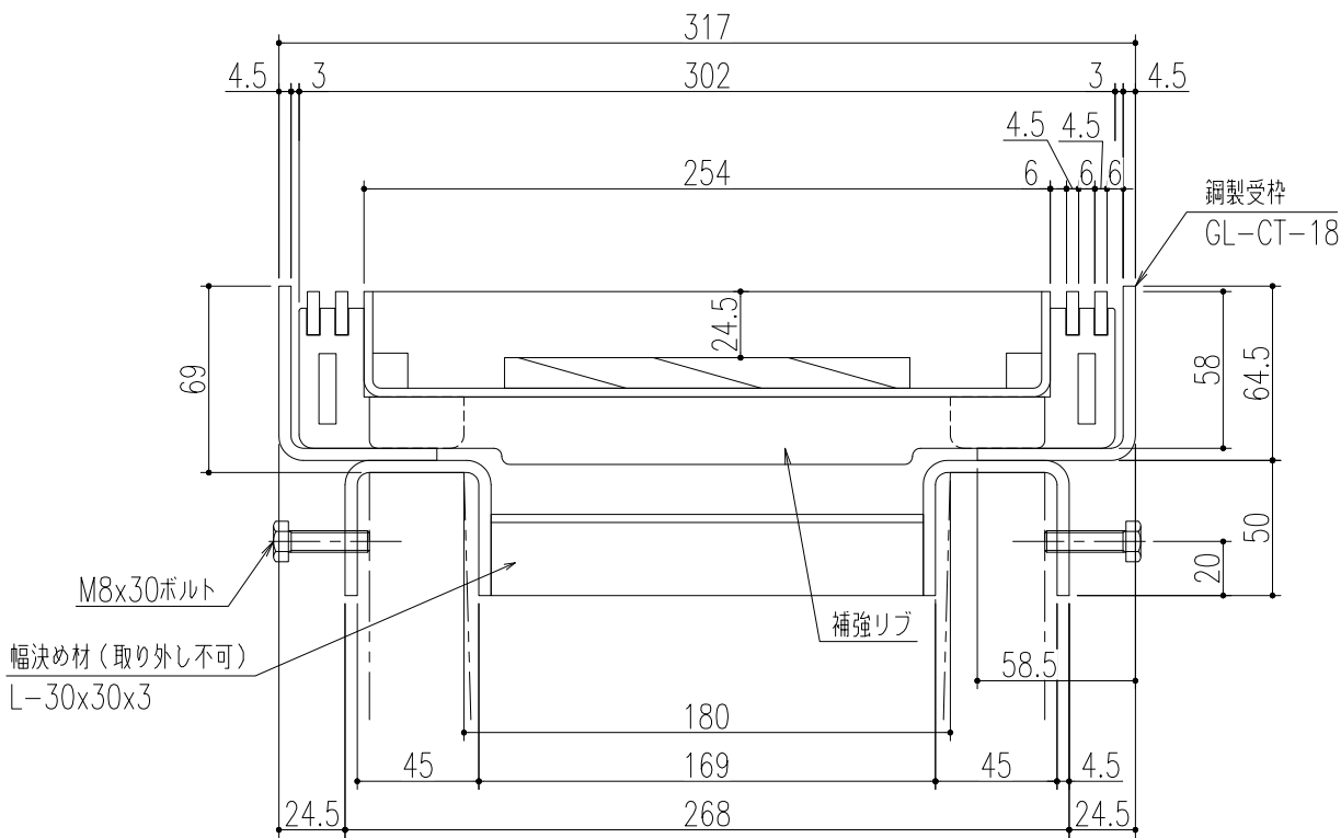
断面詳細図 S=1/3
