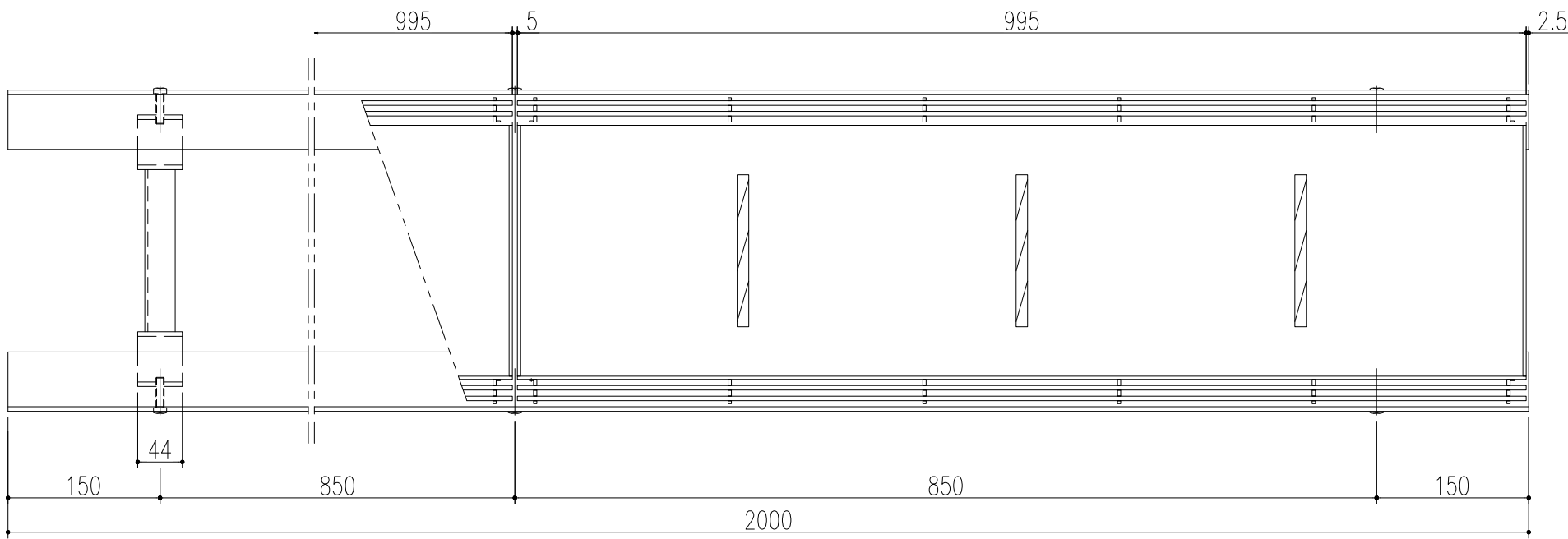
平面詳細図 S=1/6
