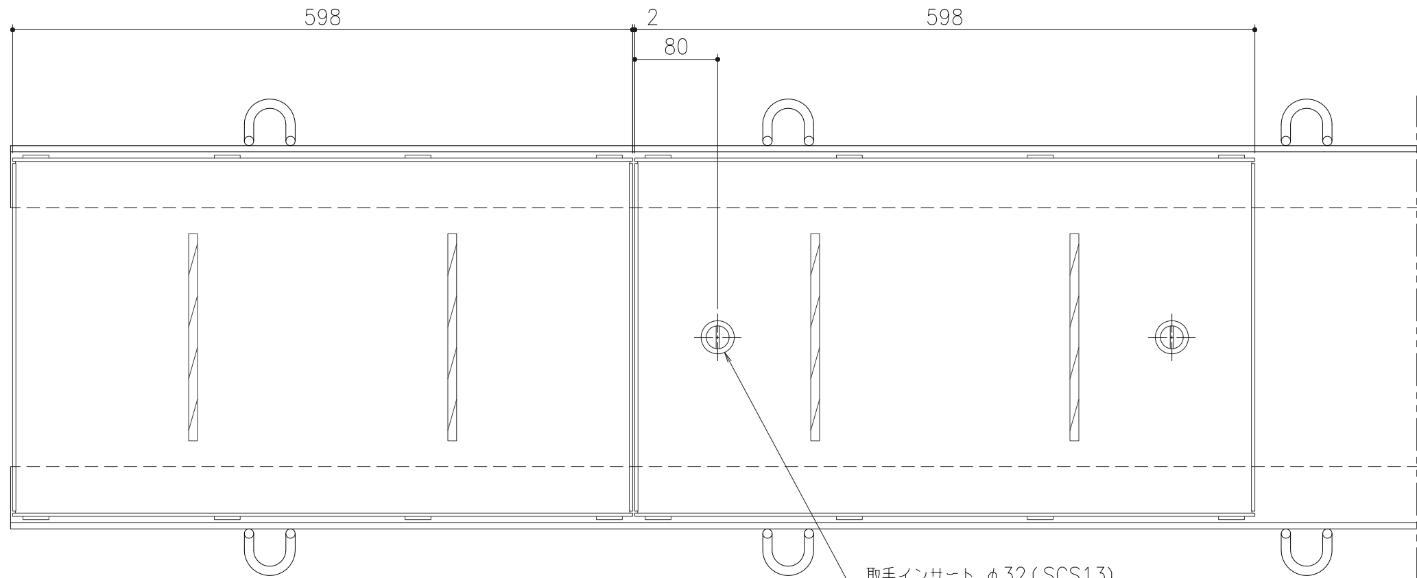
平面詳細図
