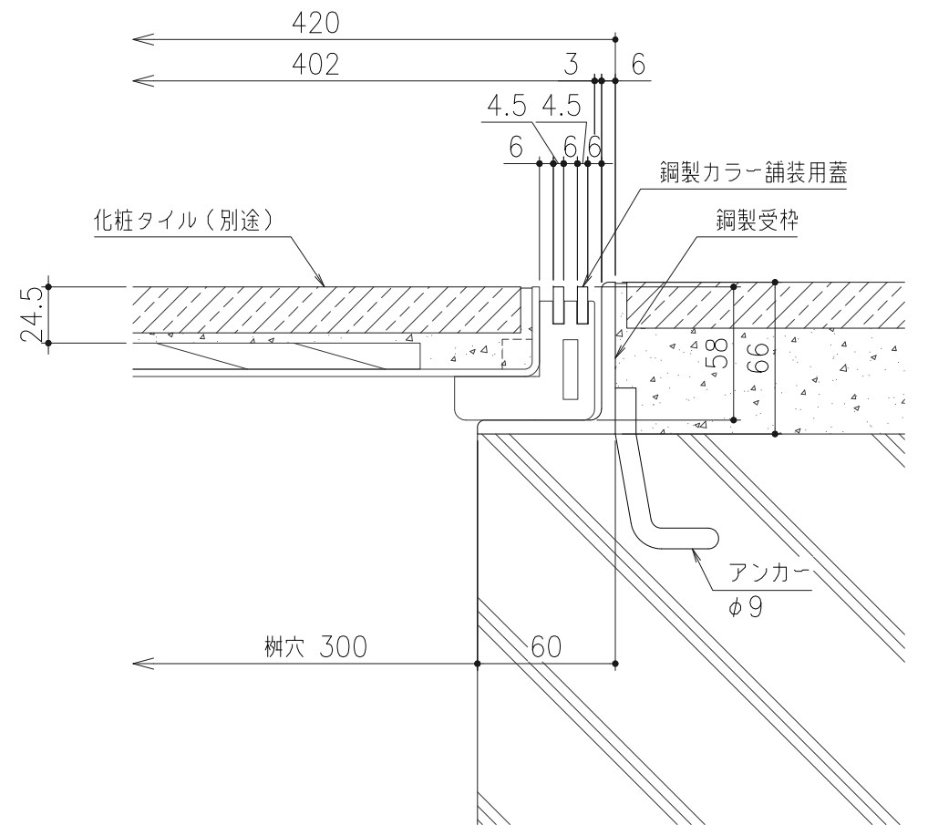
断面詳細図 S=1/3
