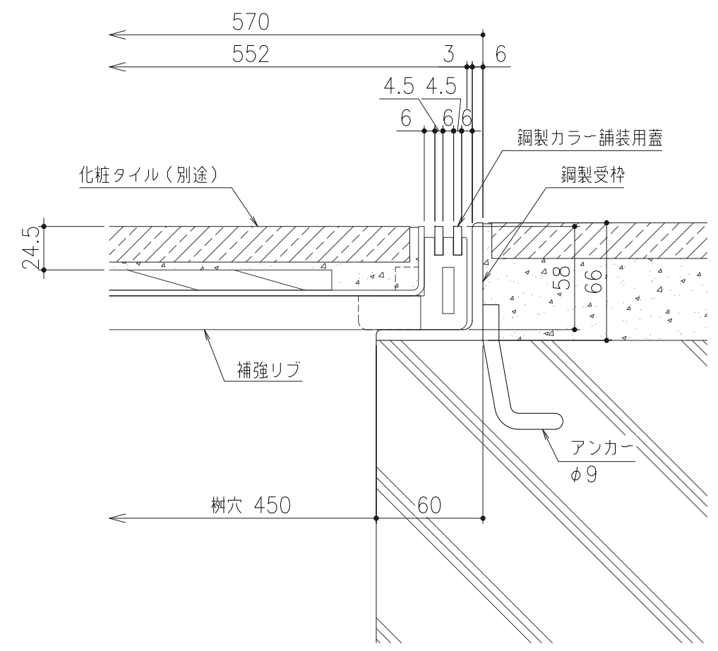
断面詳細図 S=1/3
