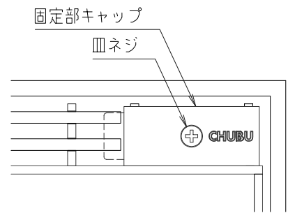
ボルト固定部詳細図 S=1/2
