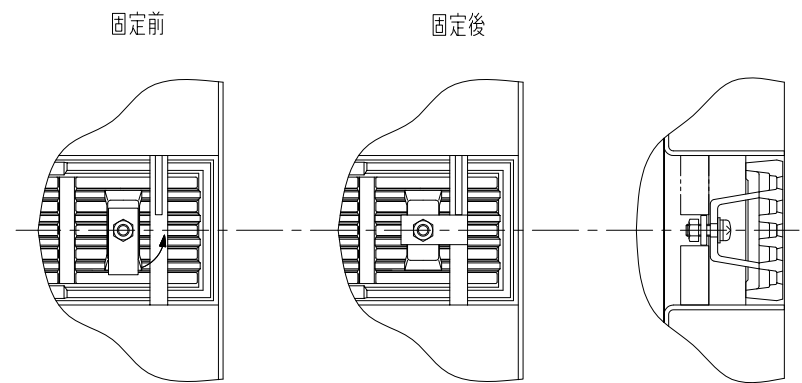
グレーチング固定部詳細図
