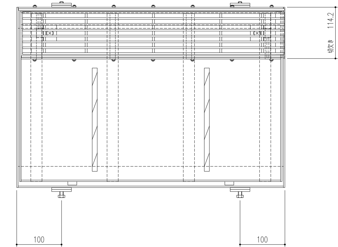
ベアリングバー詳細図
