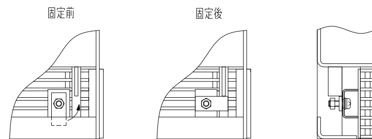
グレーチング固定部詳細図
