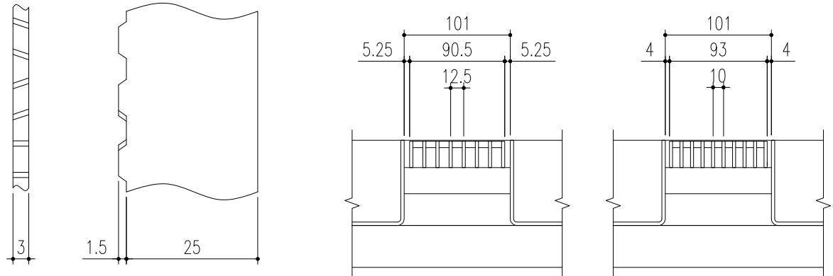
ベアリングバー詳細図
