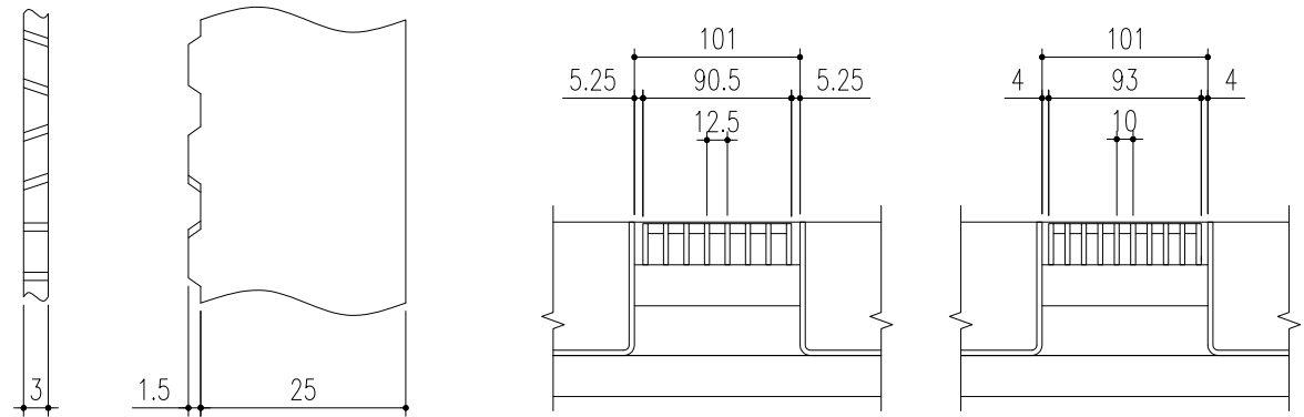
ベアリングバー詳細図
