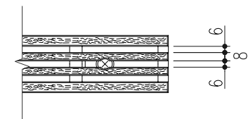
蓋詳細圖
