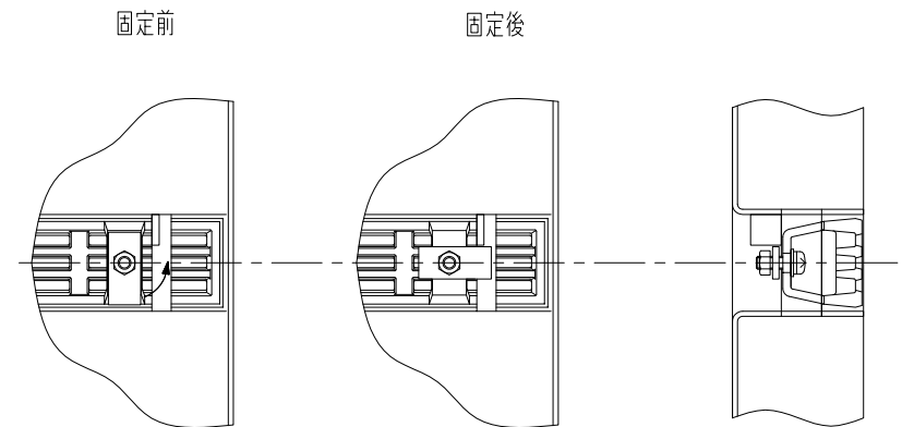
グレーチング固定部詳細図
