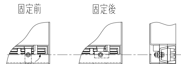
グレーチング固定部詳細図
