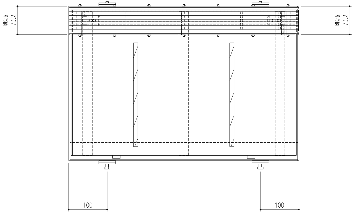
ベアリングバー詳細図
