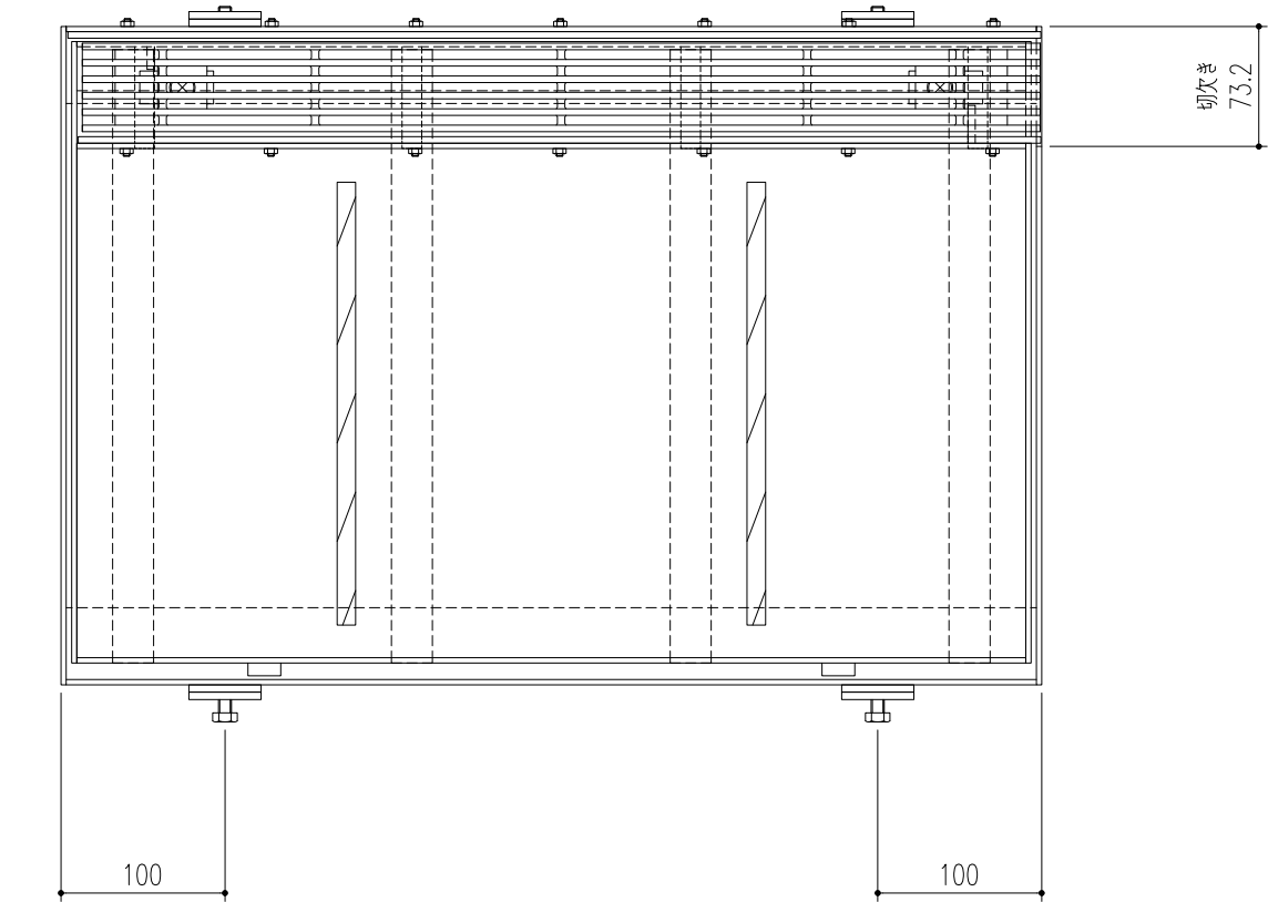
ベアリングバー詳細図
