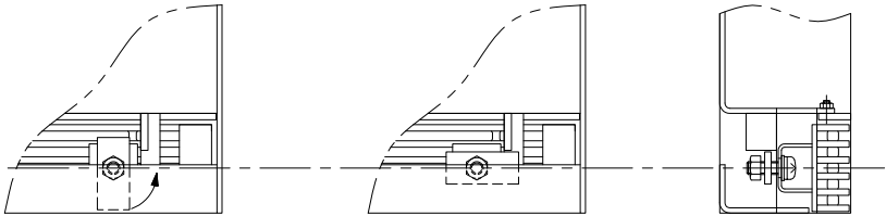
グレーチング固定部詳細図
