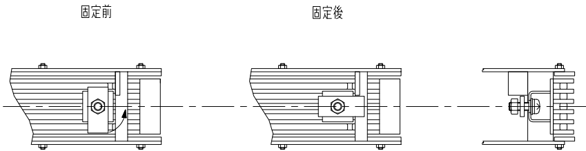
グレーチング固定部詳細図
