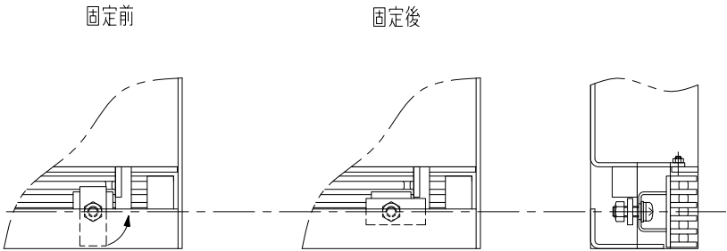
グレーチング固定部詳細図
