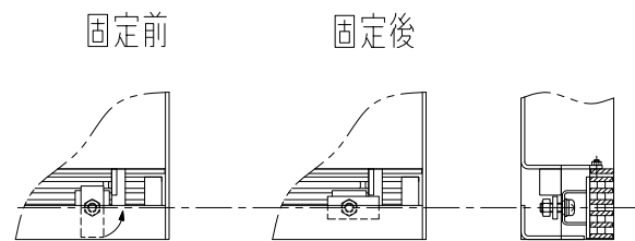
グレーチング固定部詳細図
