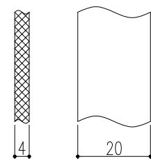
ベアリングバー詳細図
