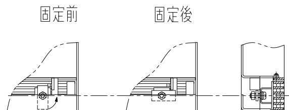
グレーチング固定部詳細図
