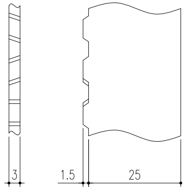
ベアリングバー詳細図
