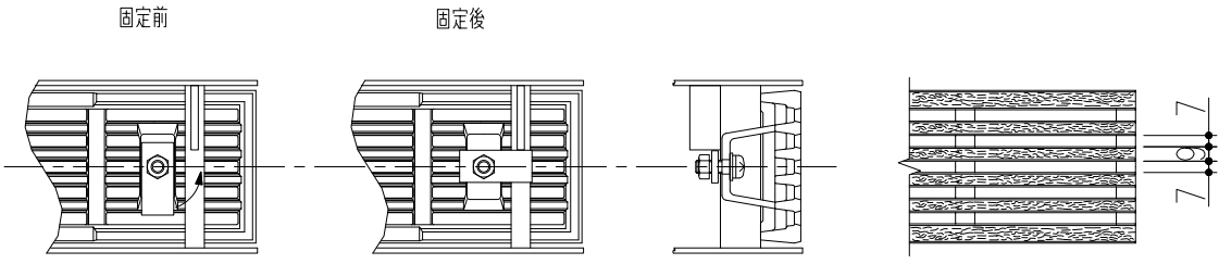
蓋詳細図
